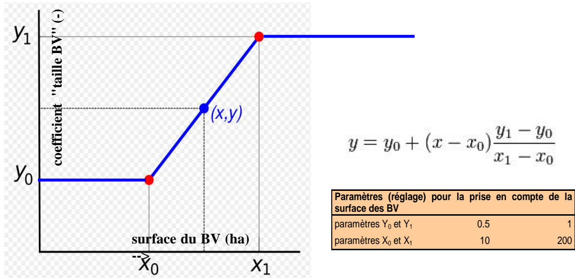
Figure 1. Calcul du coefficient Y pour la prise en compte de la taille du bassin versant.
